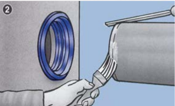
2. Зніміть фаску з кромки сполучної труби і змастіть її змаскою
