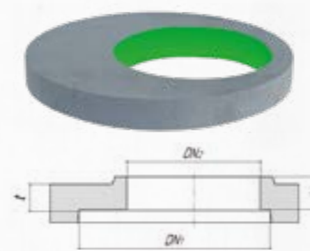
Починаючи з діаметрів 1500 можливо виготовлення плит з додатковим отвором
