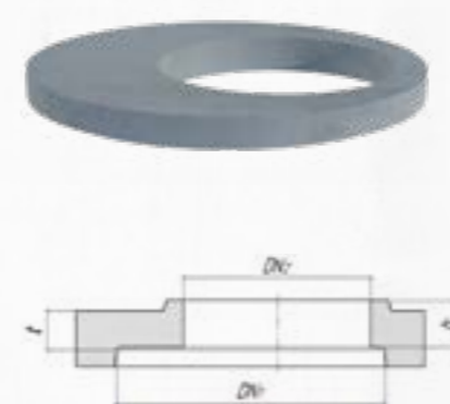
Починаючи з діаметрів 1500 можливо виготовлення плит з додатковим отвором
